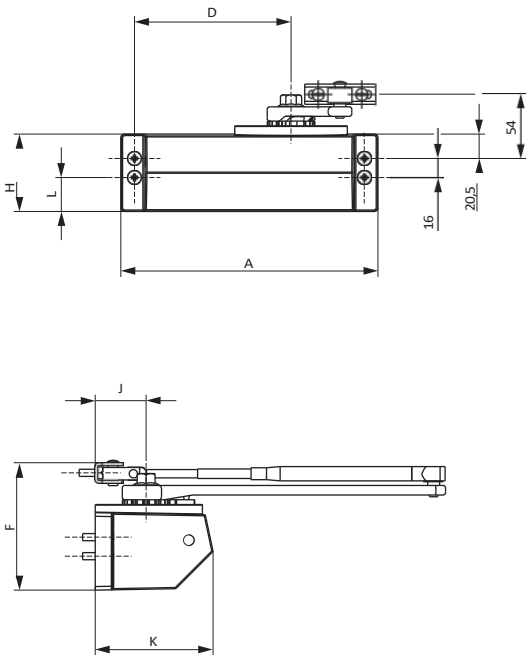
Dimensiones en función de la fuerza de cierre
